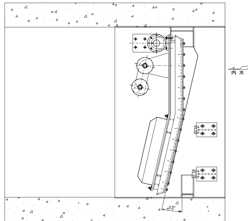
A-A(初期開度) S=1:10
