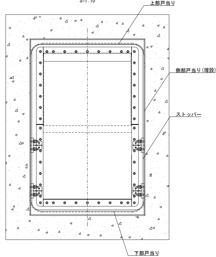
背面図 S=1:10
