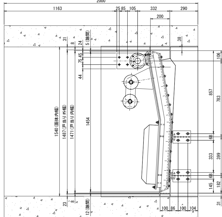
A-A(全閉時) S=1:10 2000
