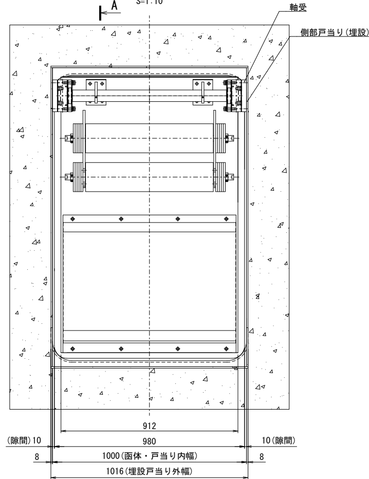
正面図 S=1:10
